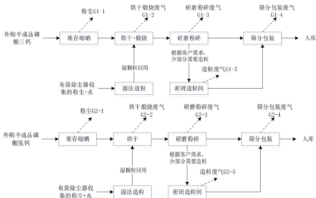
图 2-2 生产工艺及产污环节图
