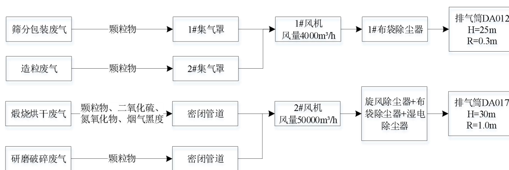
图 3-1 废气产生处理流程示意图
