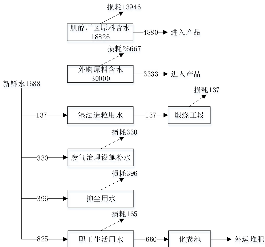
图 2-1 项目建成后全厂水平衡图 (m³/a)
